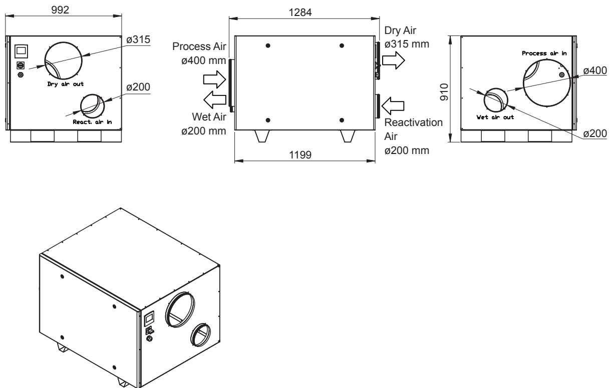
Fig. 4: Dimensions DA 500-4000
